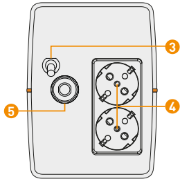
Arka Görünüş
